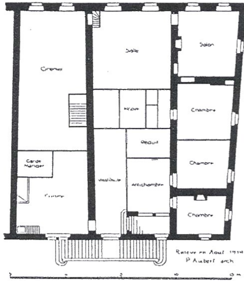
Le château. — Façade côté cour et plan du 1 er étage.
